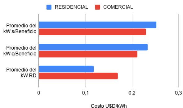
Fig. 2. Comparativa de la paridad de red en usuarios residenciales y comerciales, aplicando el beneficio y no haciéndolo.
