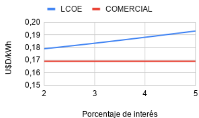
Fig. 4. Valor de LCOE con variación del porcentaje de interés (Instalación de 10 kW)
