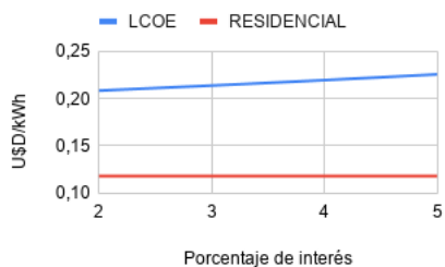
Fig. 3. Valor de LCOE con variación del porcentaje de interés (Instalación de 2 kW)
