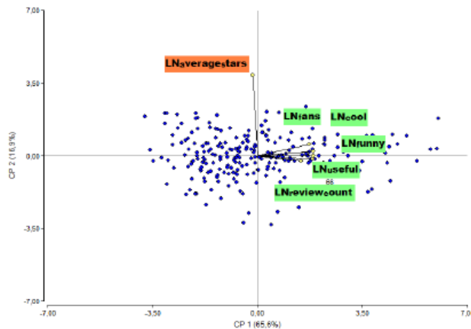
Figura 3. Gráfico biplot
