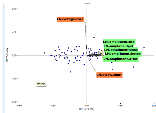
Figura 5. Gráfico biplot
